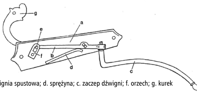
Schemat konstrukcyjny zamka lontowego z XVI wieku
